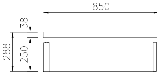
Zij aanzicht
